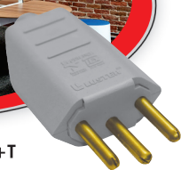
Plugue Macho 2P+T - BCO 10 A / 250 V~
